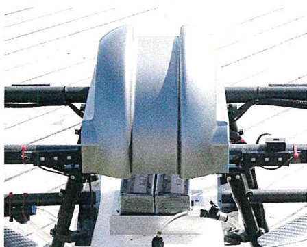
散布用ドローン専用機体カバー
